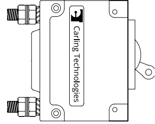
SAĞ YAN GÖRÜNÜM RIGHT SIDE VIEW
