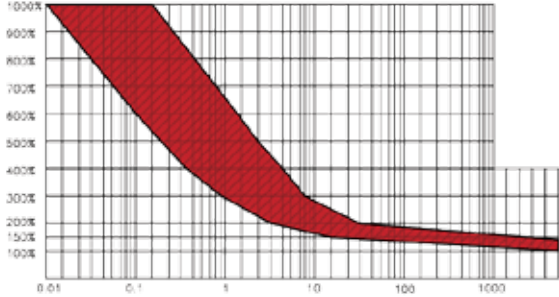
Açma Eğrisi Zaman Gecikmeli - Time Delay
